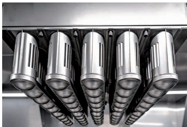
Kaseta filtrów JCE.
