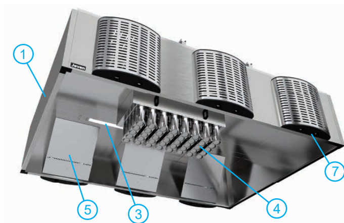
Widok okapu z dołu
