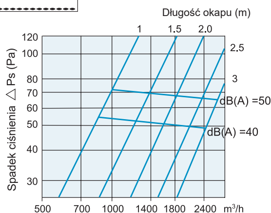
Przegrody na skropliny model 2/1
