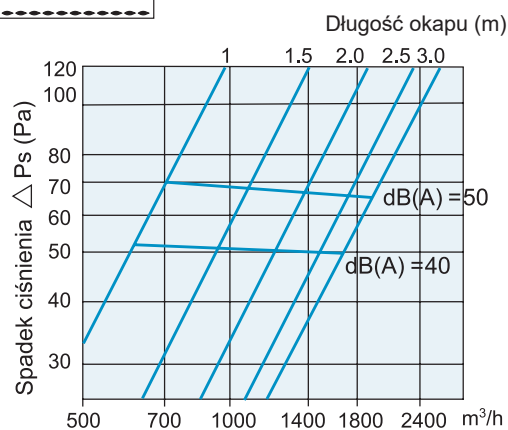
Przegrody na skropliny model 1/1
